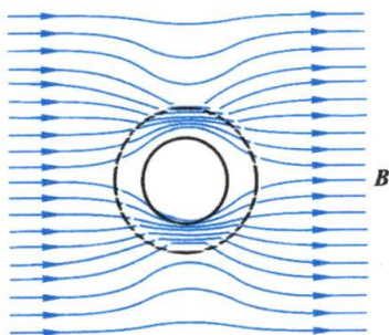
图 8-60 磁屏蔽
