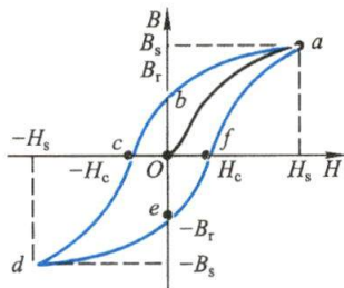
图 8-54 磁滞回线
