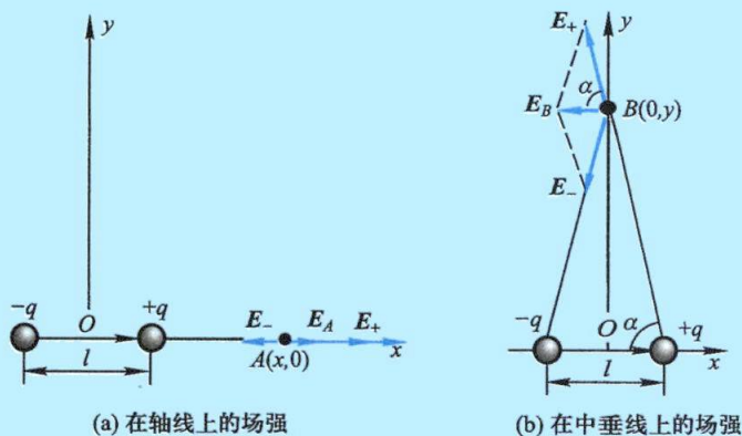
图 7-8 电偶极子
