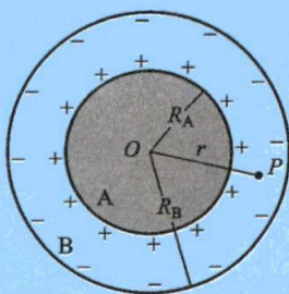
图 7-50 球形电容器
