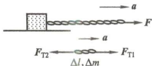
图 1-24 绳中的张力
