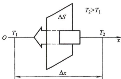
图 5-11 热传导现象
