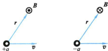
(a) \mathbf{B} 垂直于纸面向外 (b) \mathbf{B} 垂直于纸面向内
