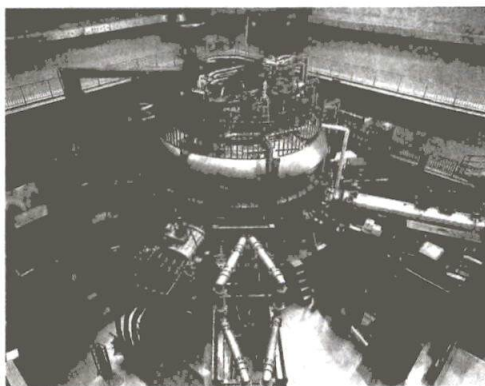
图 8-34 托卡马克
