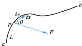
图 2-20 变力的功
