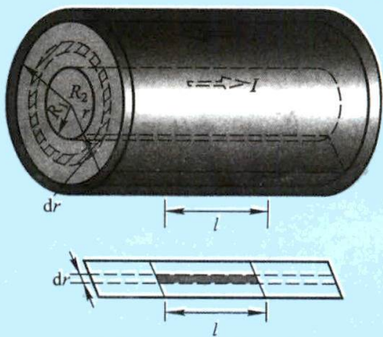
图 9-24 电缆的自感
