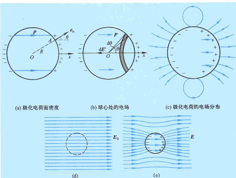
图 7-64 电介质球
