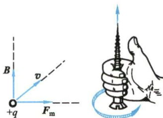
图 8-8 B 、 F_m 、 v 的方向关系
