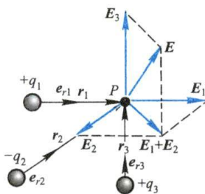
图 7-7 点电荷系的电场强度
