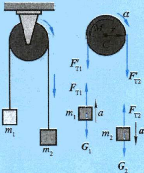
图 3-9 阿特伍德机
