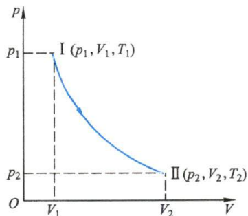
图 5-1 平衡态和准静态过程的示意图
