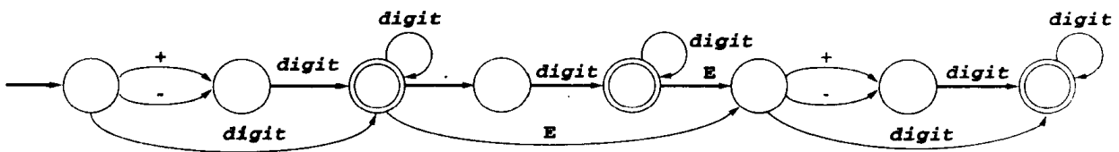
图2-3 浮点数的有穷自动机
