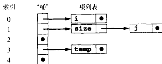
图6-11 分离链接的杂凑表,显示如何解决冲突
