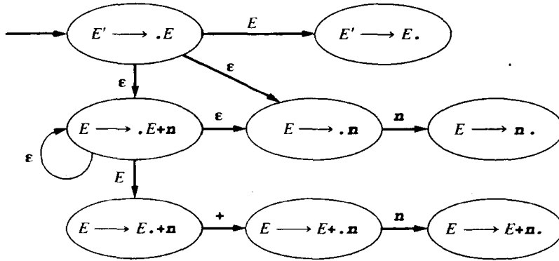
图5-2 例5.6中文法的LR(0)项的NFA
