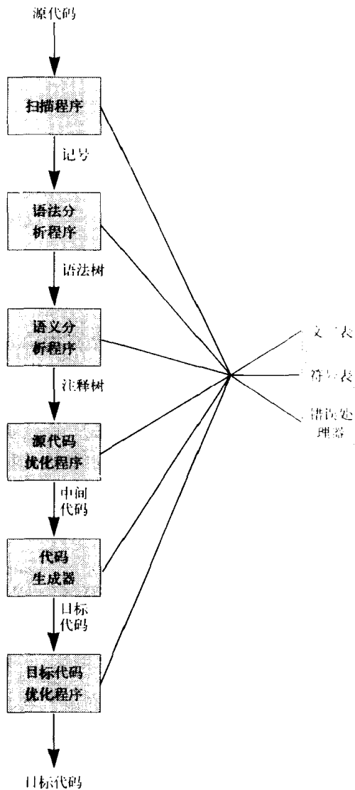
图1-1 编译器的阶段
