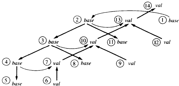
图6-7 字符串3450的相关图(例6.9)
