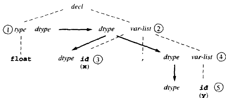
图6-9 显示例6.12遍历顺序的分析树
