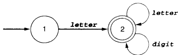
图2-1 标识符的有穷自动机
