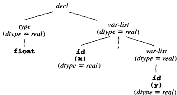
图6-3 字符串 \text{float x,y} 的语法树,显示表6-3中属性文法指定的 \text{dtype} 属性
