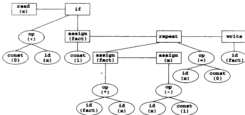
图3-6 程序清单3-3中TINY程序的语法树
