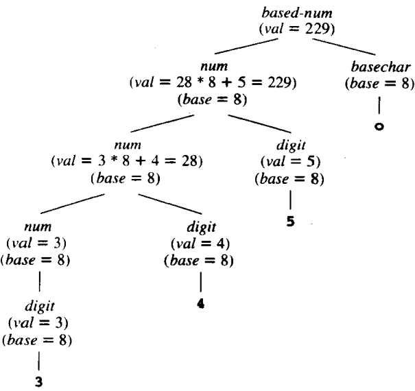
图6-4 例6.4中属性计算的语法树
