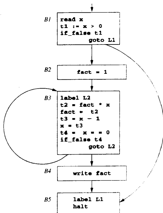
图8-4 程序清单8-2中间代码的流图
