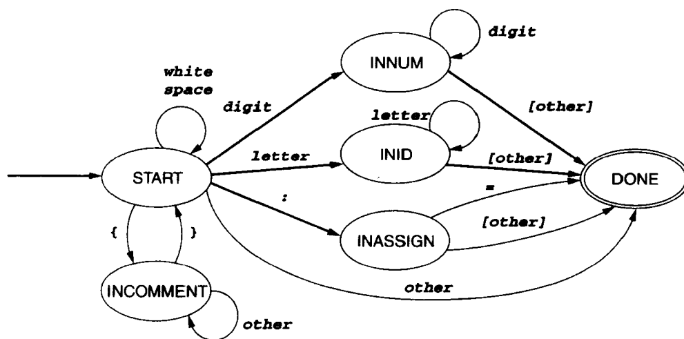
图2-8 TINY扫描程序的DFA
