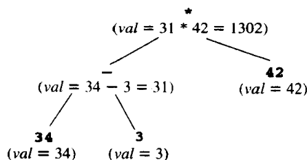
图6-5 (34-3)*42 的抽象语法树,显示表6-2或表6-5中属性文法的 val 属性计算
