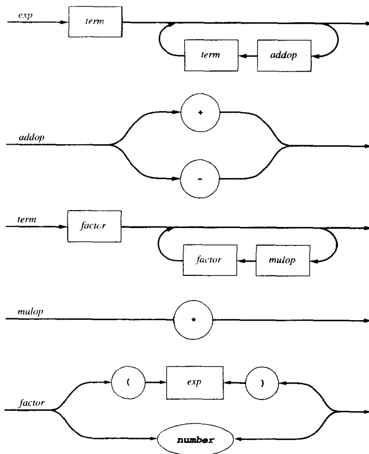
图3-4 例3.10中文法的语法图
