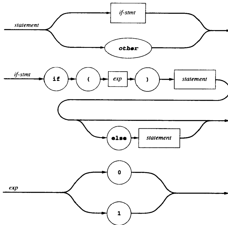
图3-5 例3.11中文法的语法图
