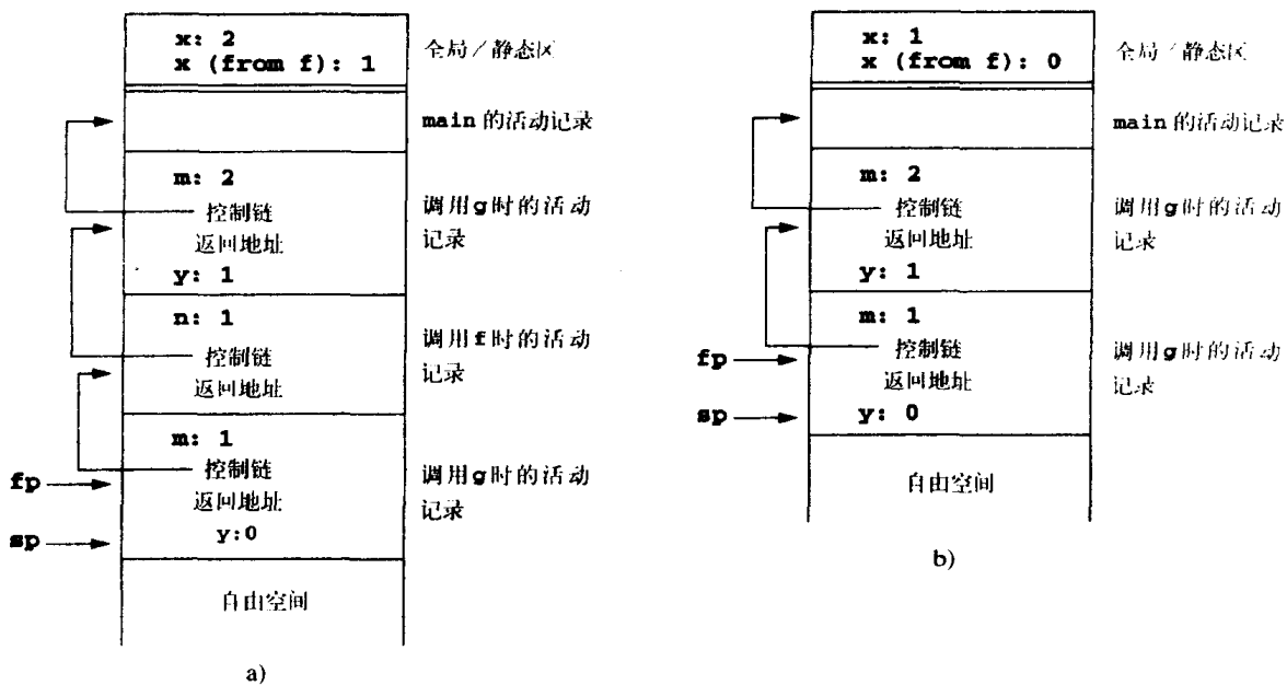
图7-3 程序清单7-3中程序的运行时环境
