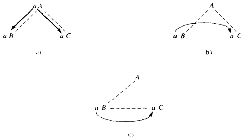
图6-8 不同种类的继承依赖
