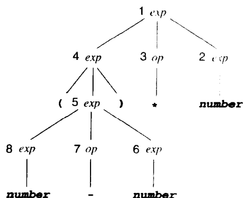
图3-3 算术表达式 (34-3)*42 的分析树
