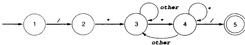
图2-4 有C风格注释的有穷自动机
