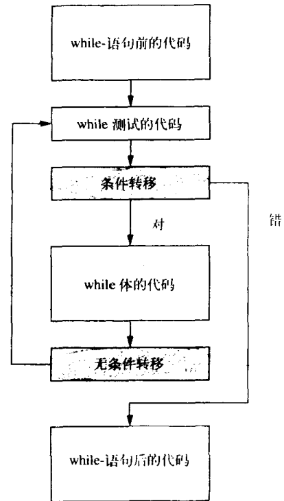
图8-2 while语句的典型代码排列
