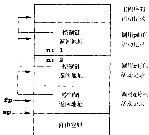
图7-5 程序清单7-4中程序的运行时栈
