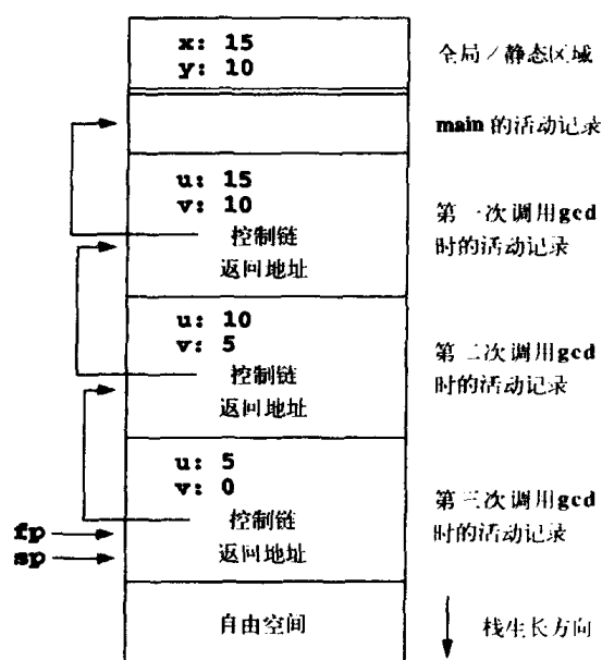
图7-2 例7.2的基于栈的环境
