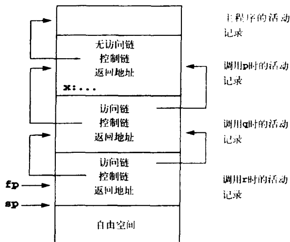
图7-7 程序清单7-5代码中第1次对 r 的调用之后的运行时栈
