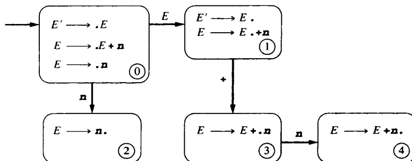
图5-4 与图5-2中的NFA相对应的项目集合的DFA
