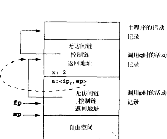
图7-9 程序清单7-6的代码中调用p之后的运行时栈
