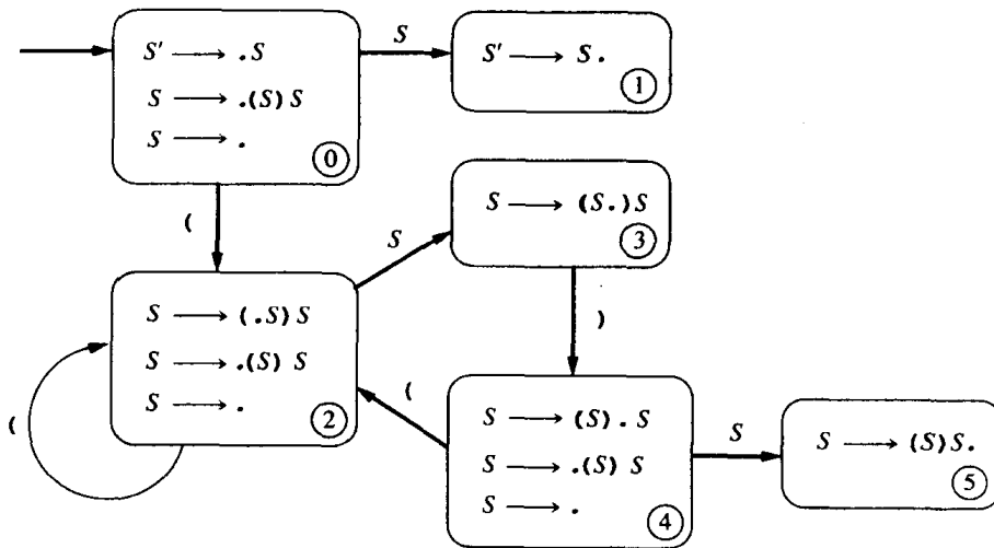
图5-3 与图5-1的NFA相对应的项目集的DFA
