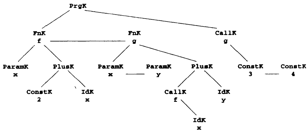
图8-3 上面程序例子的语法树
