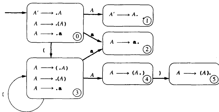
图5-5 例5.9的项目集合的DFA
