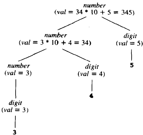
图6-1 显示例6.1中属性计算的语法树
