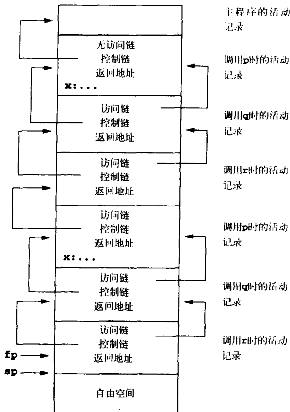
图7-8 在程序清单7-5的代码中对 x 的第2次调用之后的运行时栈
