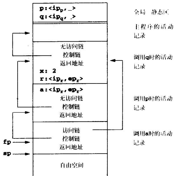
图7-11 程序清单7-6的代码调用a之后的运行时栈,所有的过程都作为环境中的闭包
