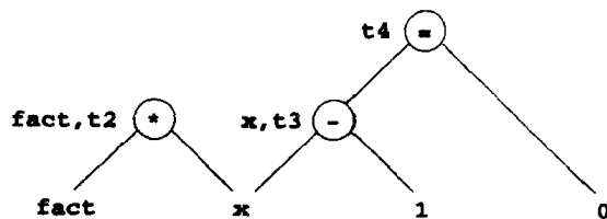
图8-5 图8-18中基本块B3的DAG
