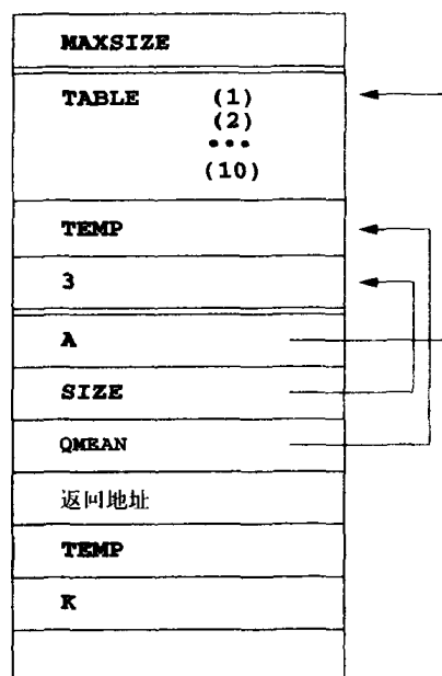
图7-1 程序清单7-1中程序的运行时环境
