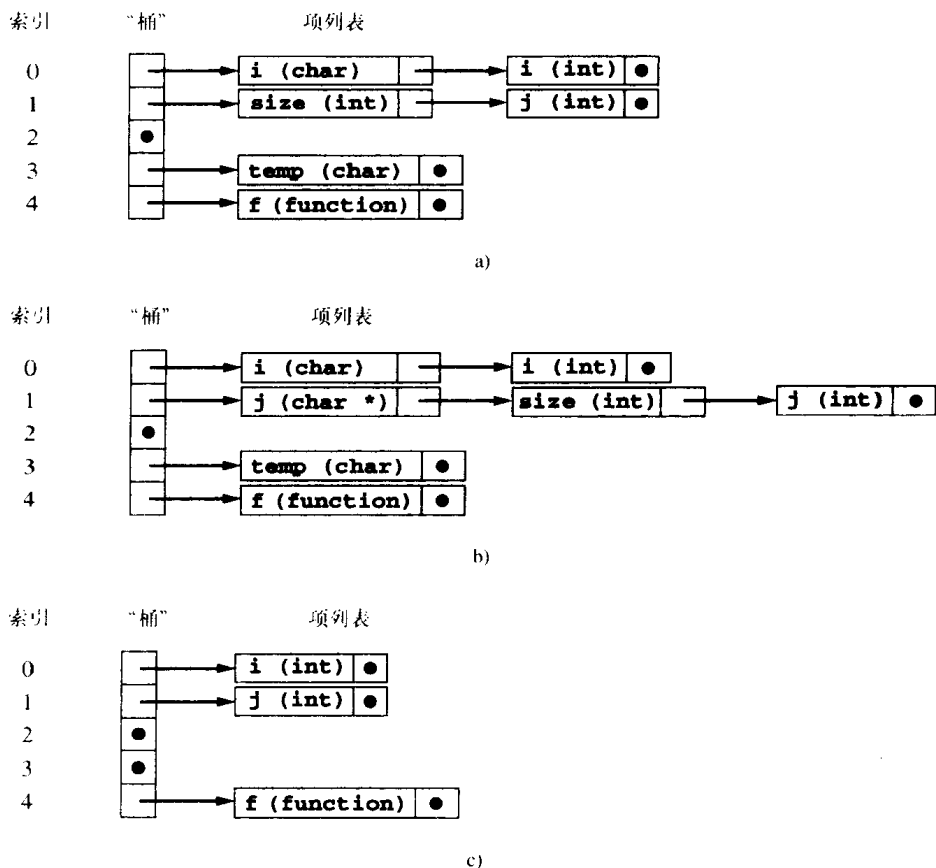
图6-12 符号表内容程序清单6-3
