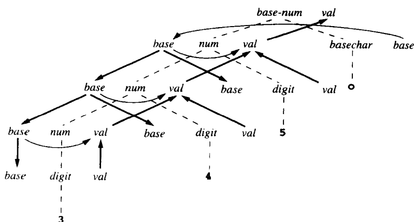
图6-6 字符串3450的相关图(例6.8)
