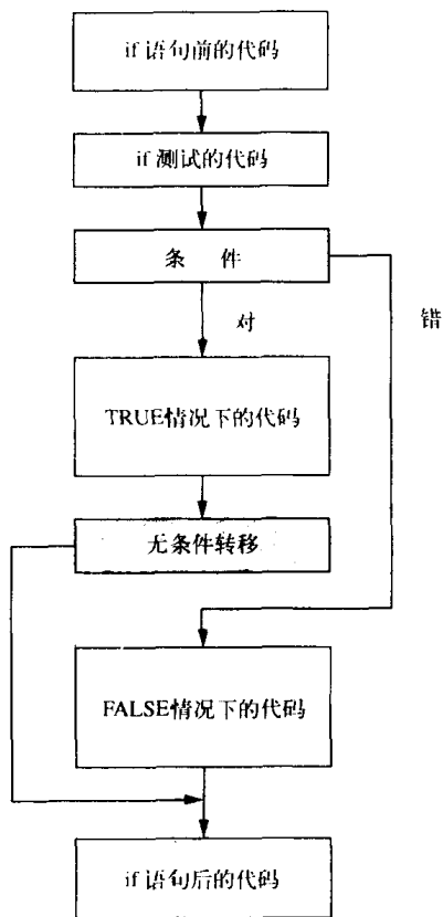
图8-1 if语句的典型代码排列
