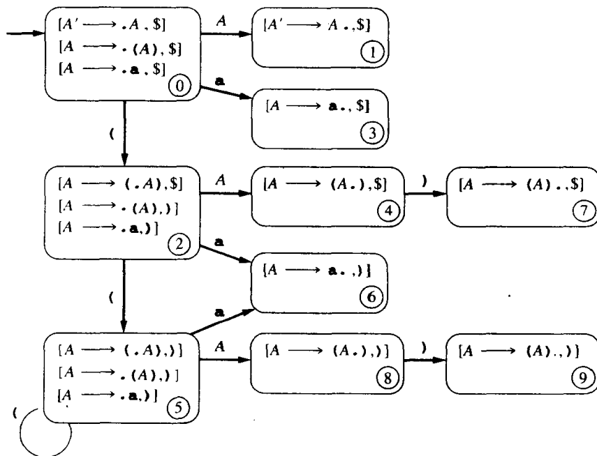
图5-7 例5.14的LR(1)项目集合的DFA
